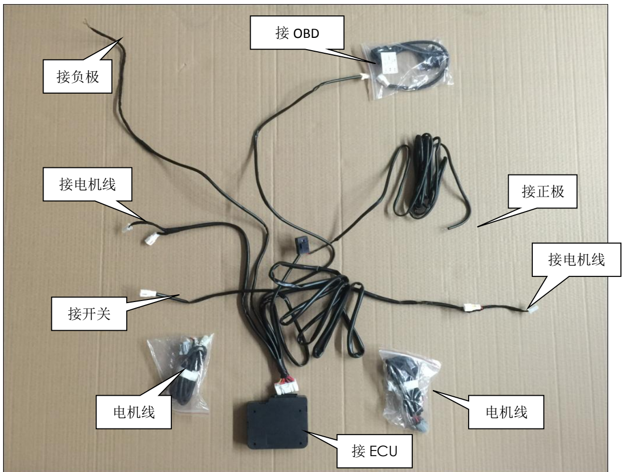
线束接线图
