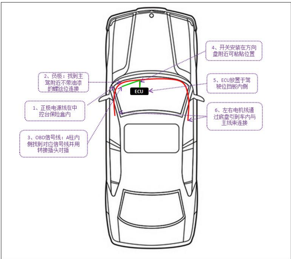
线束接线图
